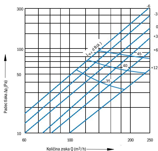
PV-2N, velikost 150
