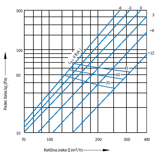
PV-2N, velikost 200
