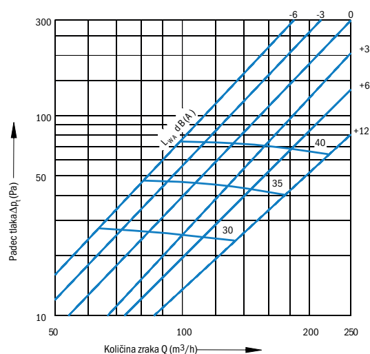
PV-2N, velikost 125
