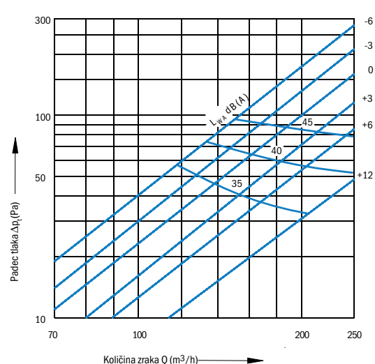
PV-2N, velikost 160
