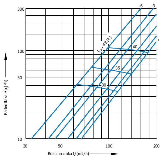
PV-2N, velikost 100
